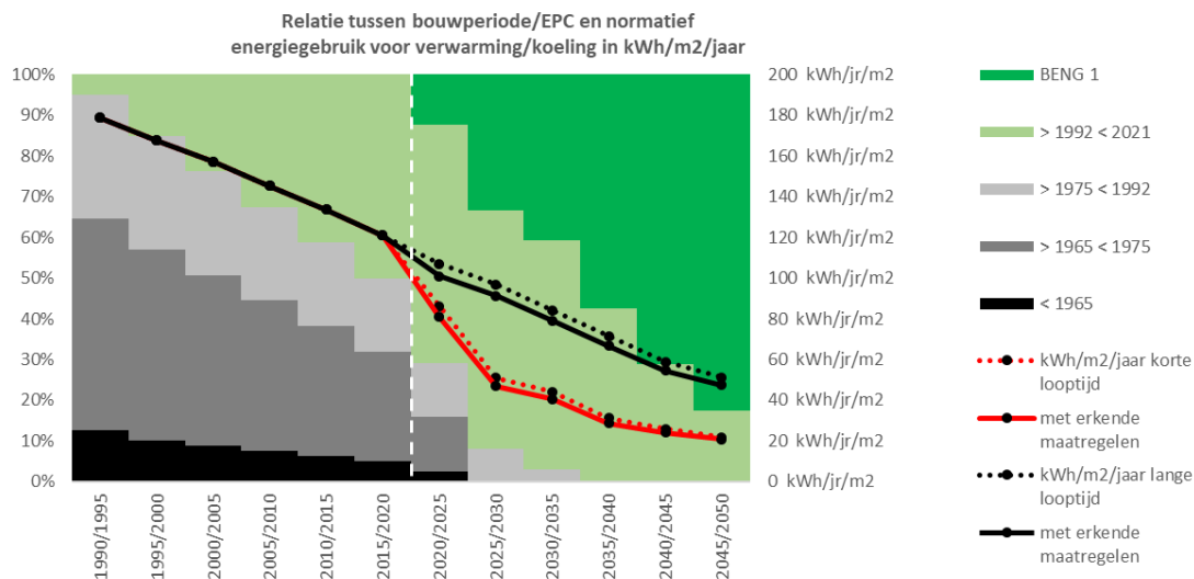
Grafiek 5: Relatie tussen bouwperiode, energievraag verwarmen en vanaf 2020 een korte exploitatielooptijd
