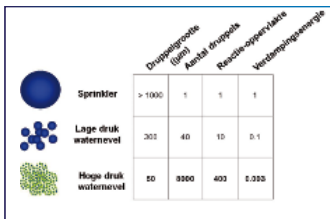
Figuur C-2: Het verschil tussen watermist- en sprinklerdruppels
