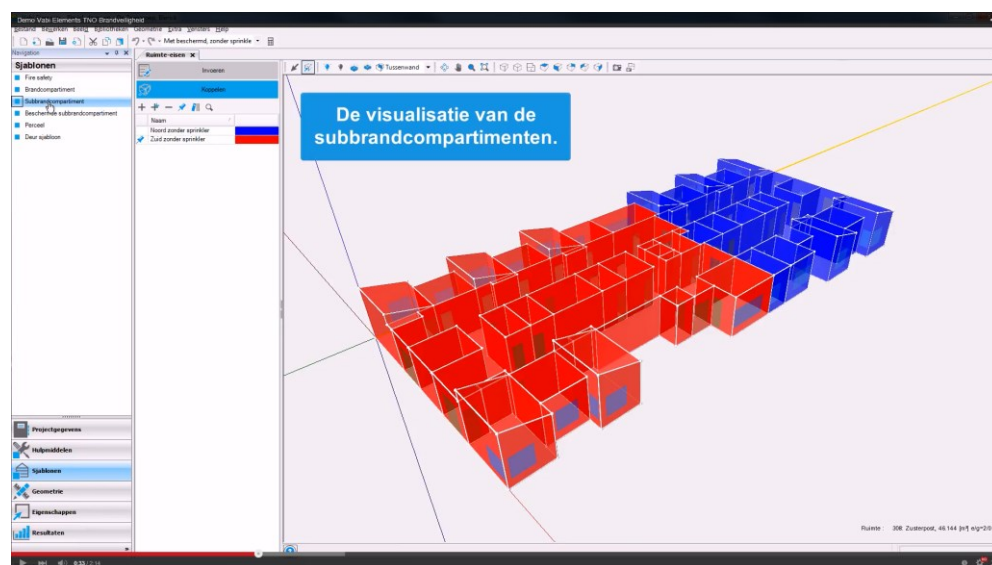
Figuur 6 Screenshot in het 3D-gebouwmodel van een plattegrond van een zorginstelling. De twee subbrandcompartimenten zijn weergegeven.
