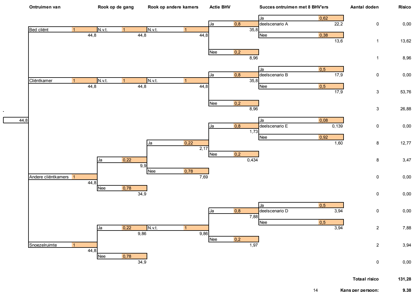
Figuur 4 Deel uitgewerkte gebeurtenissenboom (gegeven waarde voor berekende kansen en risico's vermenigvuldigen met 10^{-6} ).
